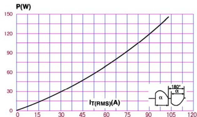
1、功耗与电流曲线 (180°C)
