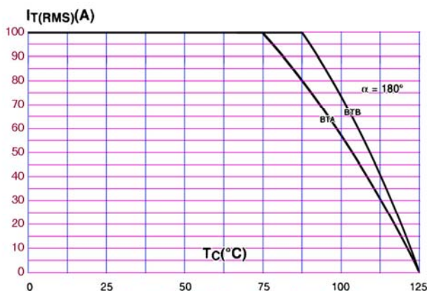
2、壳温与通态方均根电流曲线
