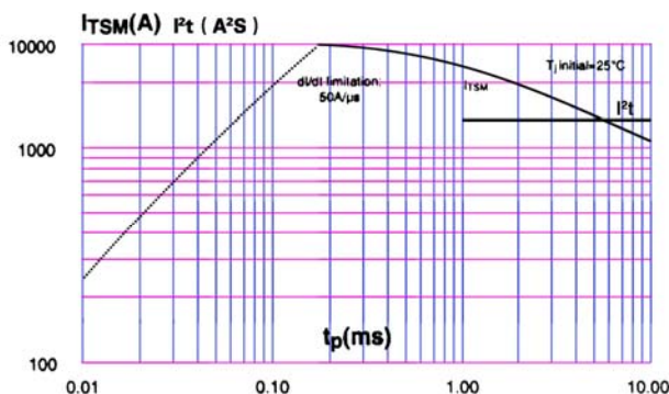
6、 I_{TSM}-t, I^2t-t 曲线
